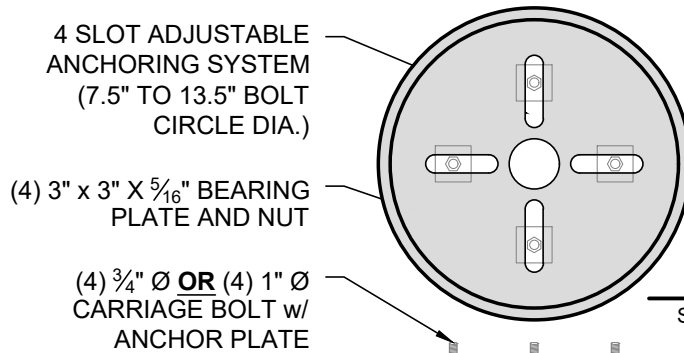
TOP VIEW SCALE: 3/4" = 1'-0"
